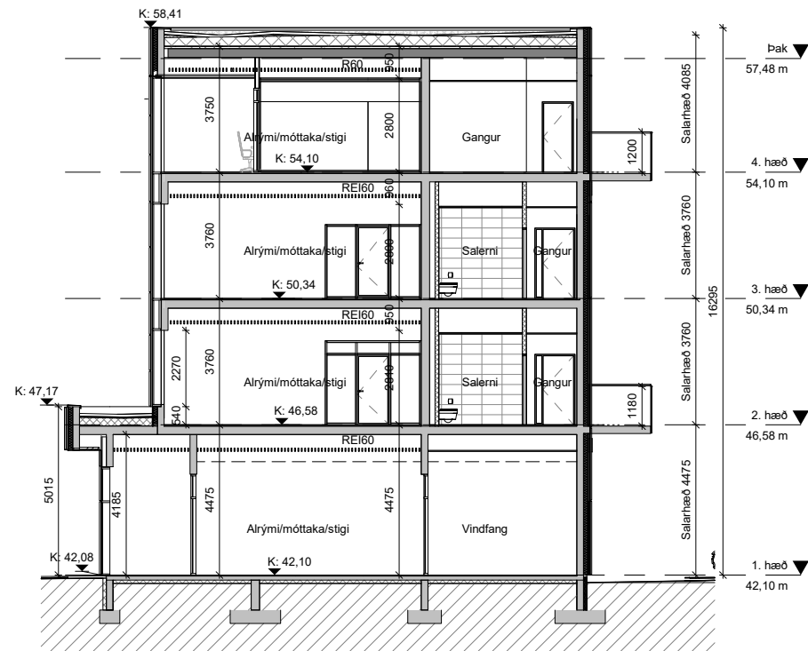
2 Snið B-B 1 : 100
