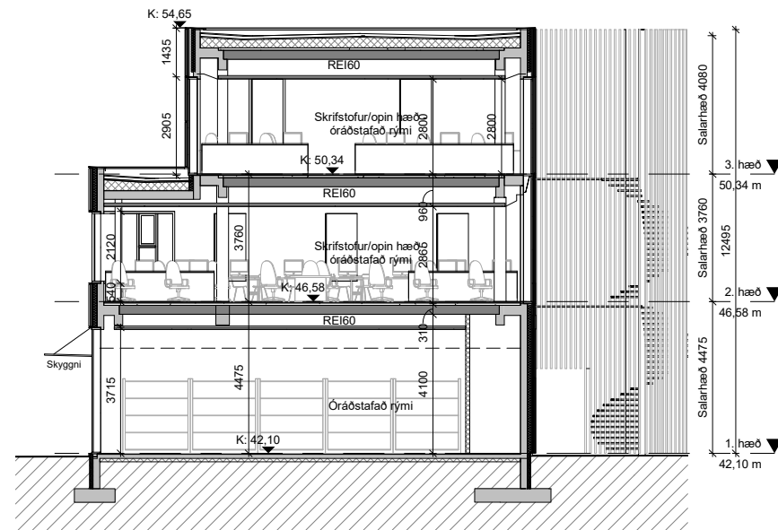
1 Snið A-A 1 : 100
