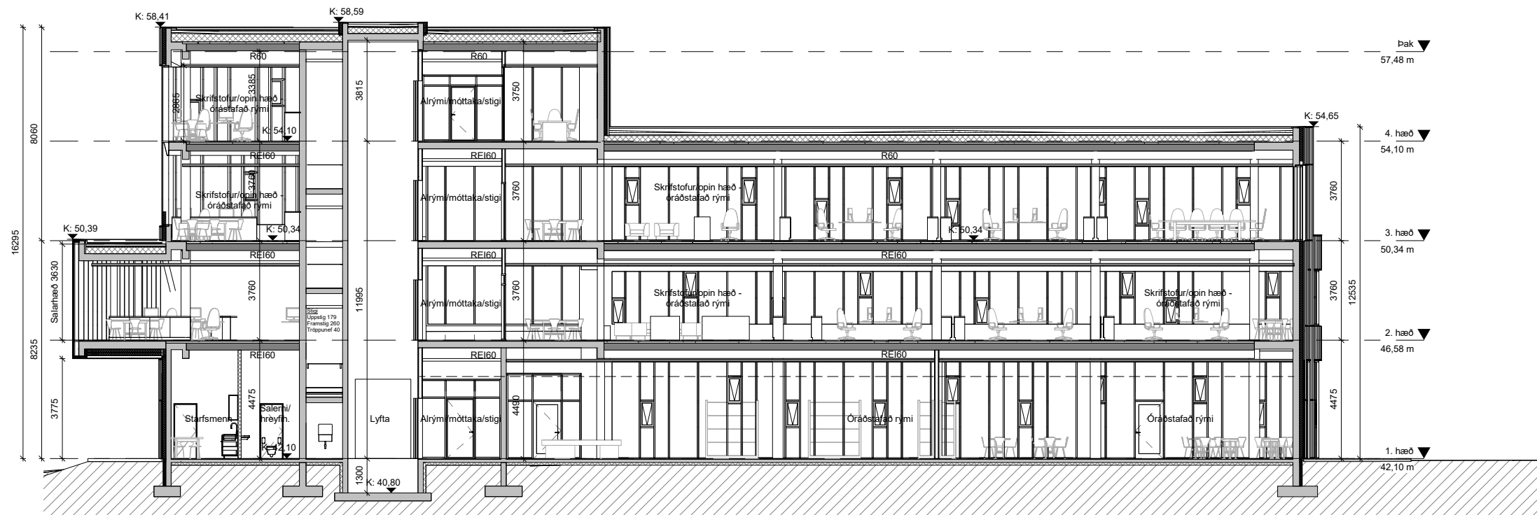
3 Snið C-C 1 : 100
