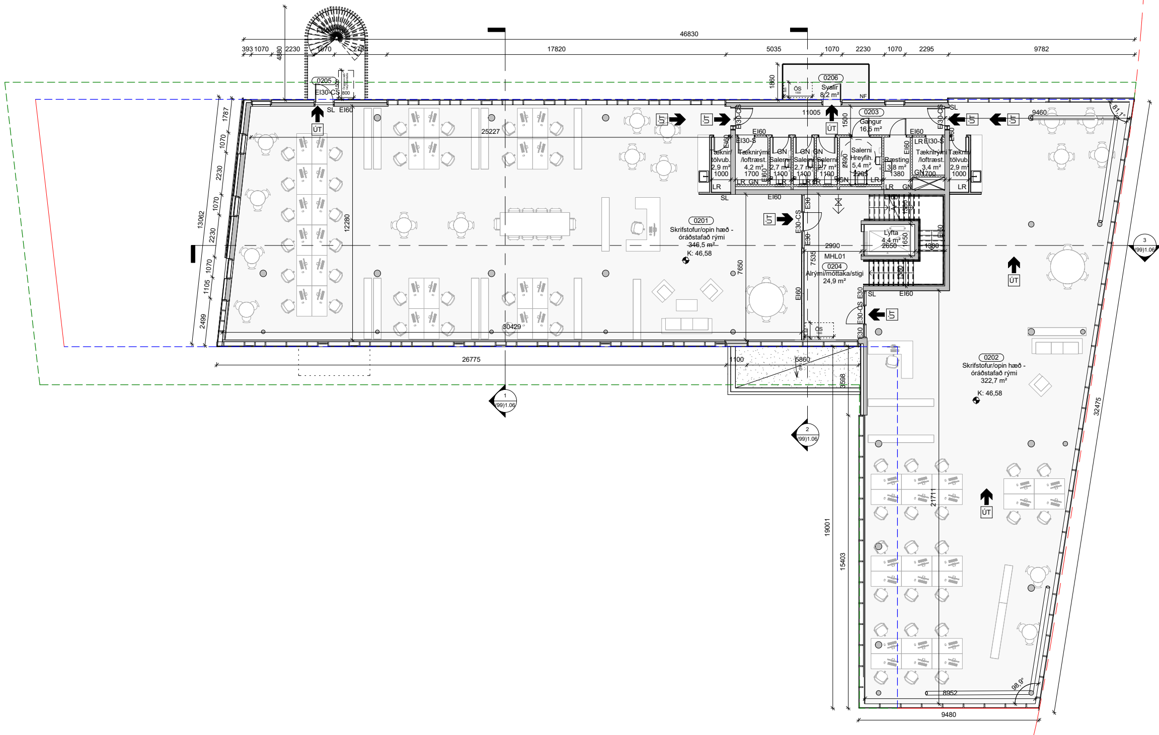
1 GRUNNMYND 2.HÆÐ 1 : 100
