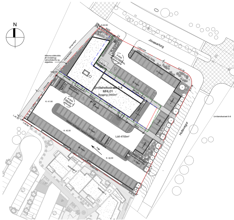
1 AFSTÖÐUMYND 1 : 500
